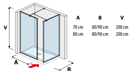
skleněné stěny / walk in do rohu pro sprchovou vaničku 70, 80 x 80 cm a 70, 80 x 90 cm
