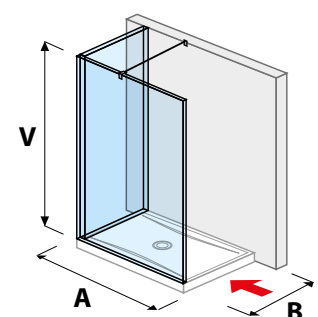
skleněná stěna PURE „L“ 120, 140 x 90 cm
