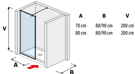
skleněná stěna boční 70, 80 cm
