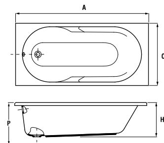
Instalační rozměry vany s panelem
