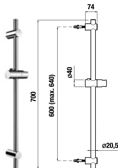
Variabilní upevnění sprchové tyče.
