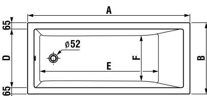
Instalační rozměry vany bez panelu
